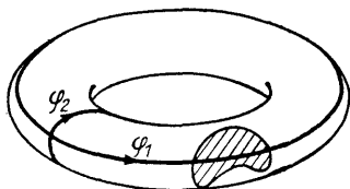
Fig. 172. The torus
