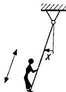
Fig. 192. A swing
