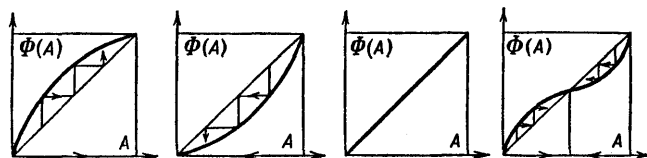
Fig. 18. Lamerey diagrams
