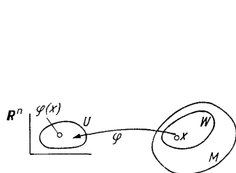
Fig. 232. A chart
